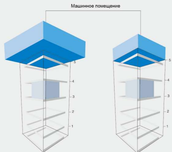
Машинное помещение в пассажирском лифте GRPS20 с небольшим машинным помещением
